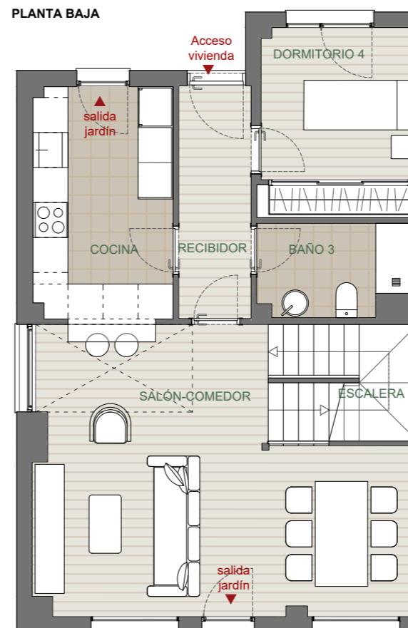
PLANTA BAJA
