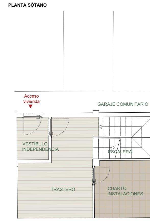
PLANTA SÓTANO
