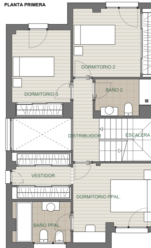
PLANTA PRIMERA
