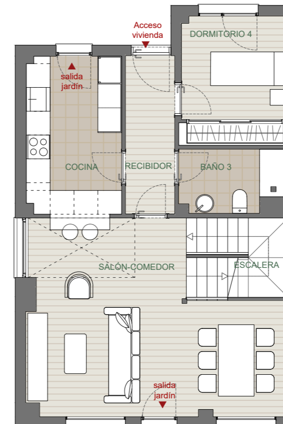
PLANTA BAJA
