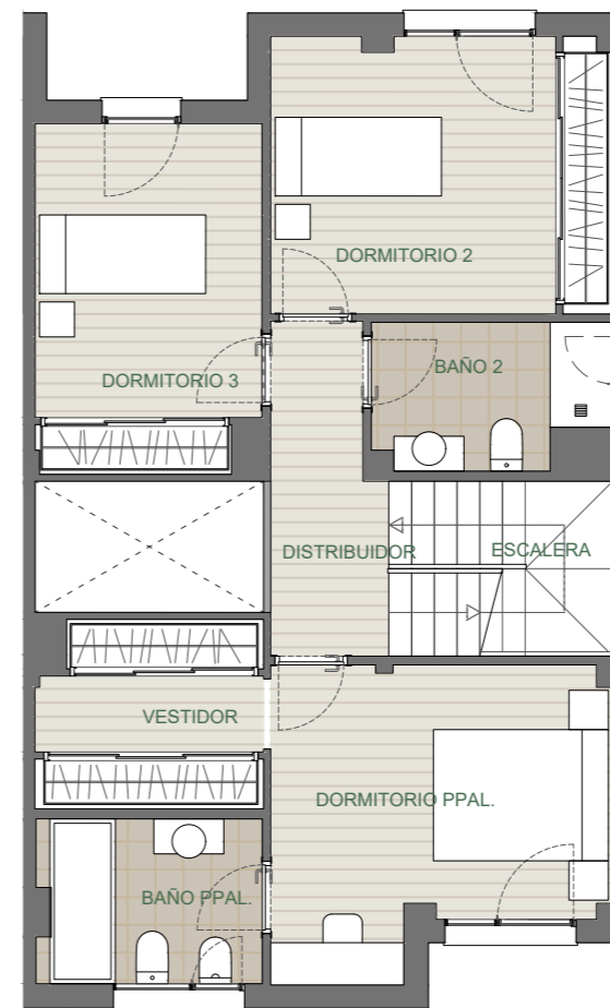
PLANTA PRIMERA
