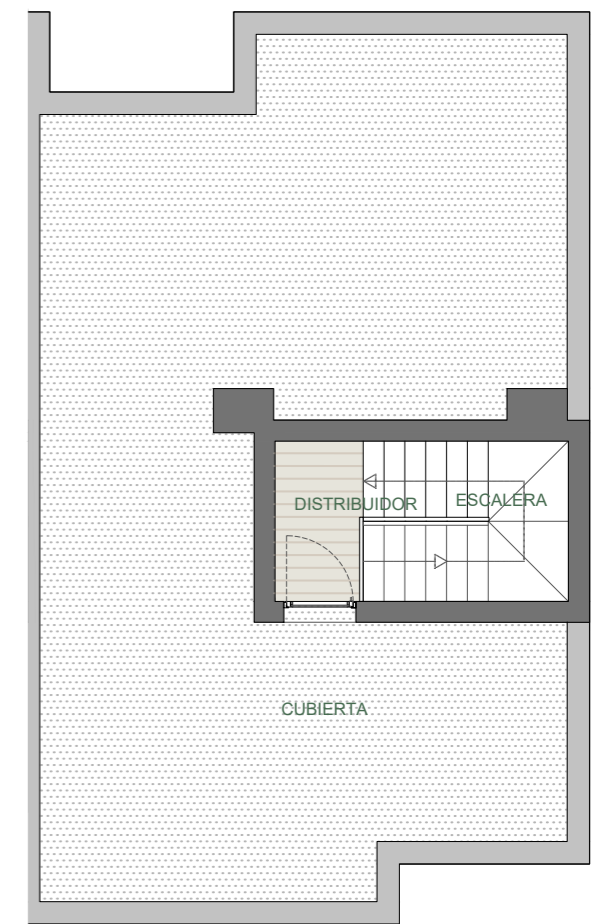
AZOTEA
