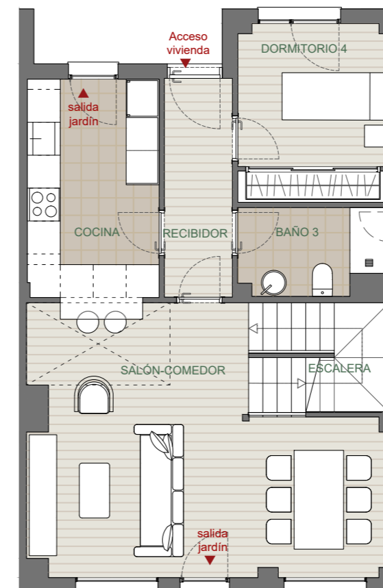
PLANTA BAJA
