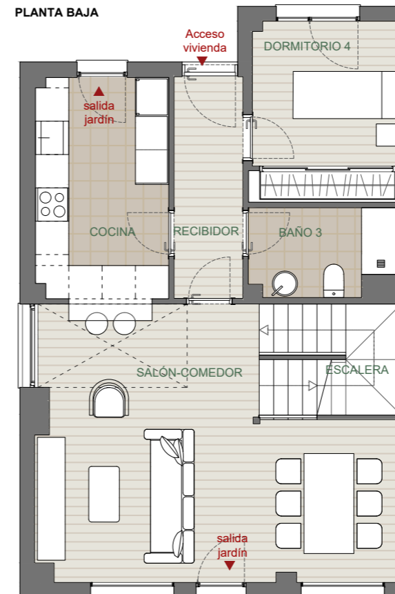
PLANTA BAJA
