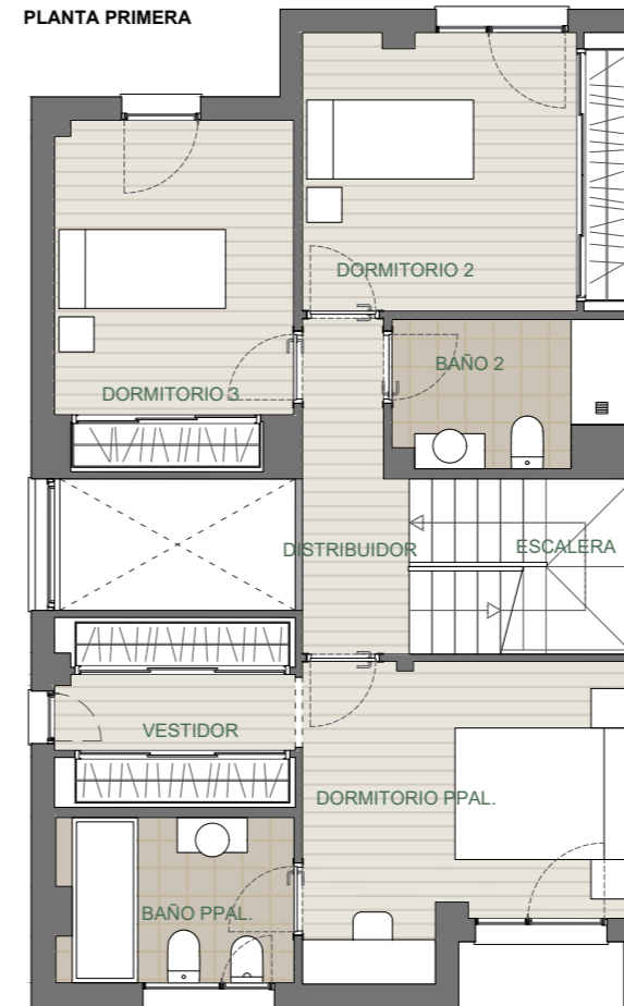
PLANTA PRIMERA
